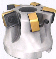
FFQ8 高送り加工用 リード角12°
